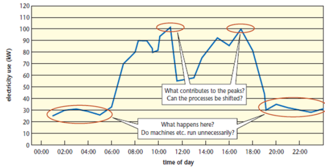
სურ. 40. ელექტრული დატვირთვის დიაგრამა
